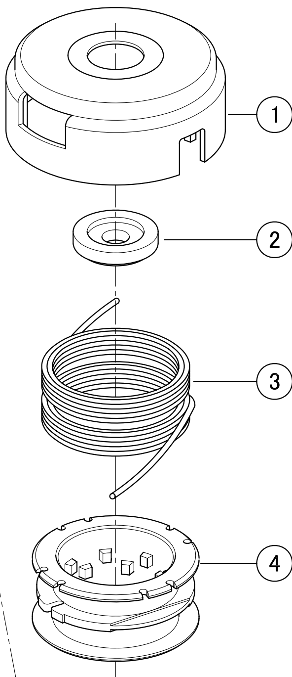
部品表
